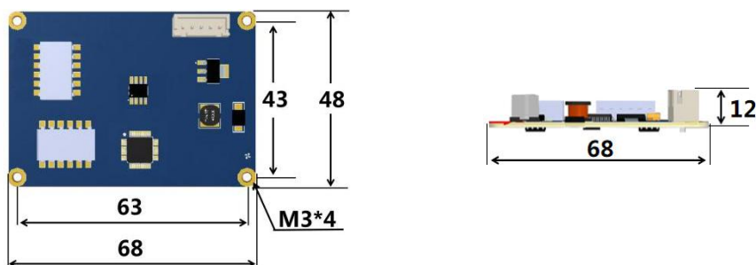
产品尺寸 L68*W48*H12mm
